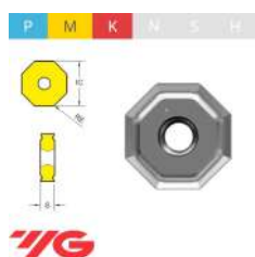
ONMU 080608 - YG602 PLACA DE FRESAR
