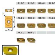
CANELA ADMW-C PLACAS DE RADIOS CONVEXOS
