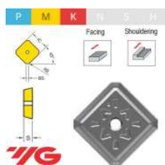
YG1 SEKR1203AFTN-YG602 PLACA DE FRESAR
