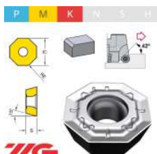
ODMW0605... PLACA DE FRESAR
