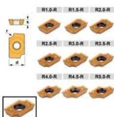
PLACAS DE FRESAR ADMT-R 1503 DE RADIO CÓNCAVO
