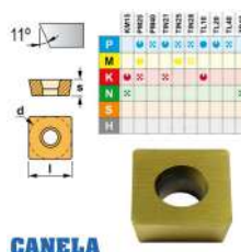
CANELA SPMW PLACA DE FRESAR
